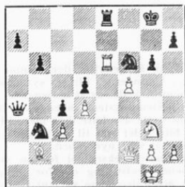
Botvinnik
