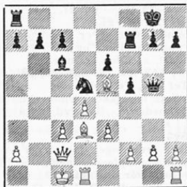
Teichmann
