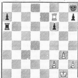
Tschigorin
